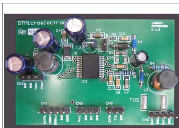
STEVAL-CBL003V1
